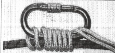
Схватывающий Бахмана
