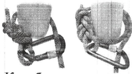
Карabinная удавка
